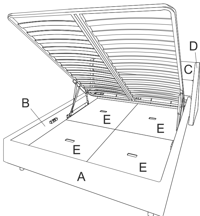
Инструкция по сборке кровати Madrid с подъёмным механизмом и бельевым ящиком
