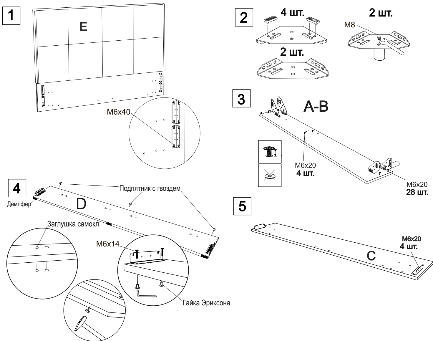
Схема установки подпятников
