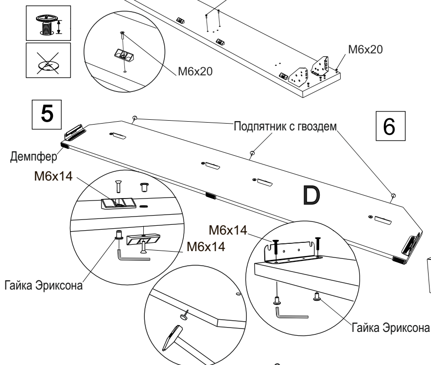
Схема установки подпятников
