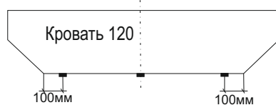
Схема установки подпятников
